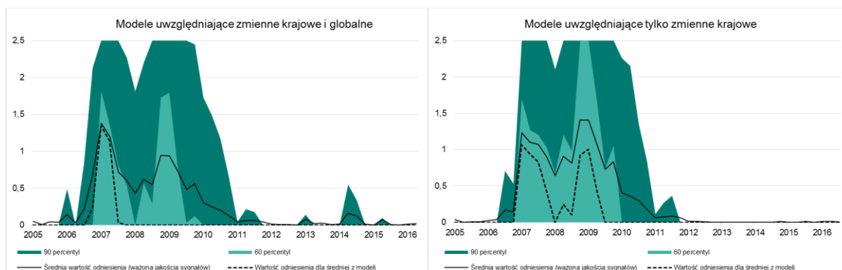
Wykres 5. Wartość bufora antycyklicznego w Polsce implikowana przez modele wczesnego ostrzegania
